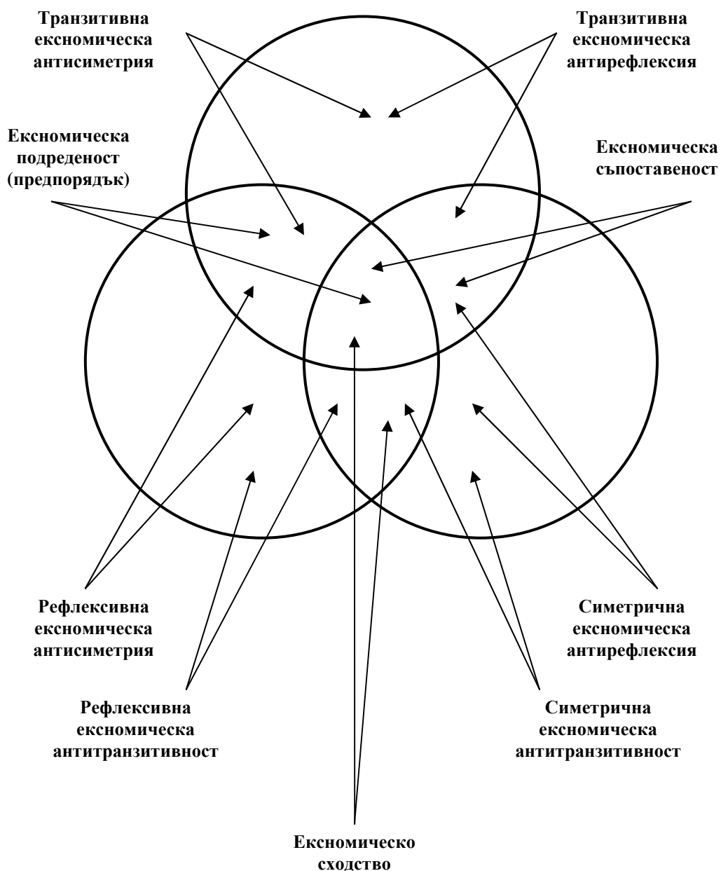
Фиг. 5.2. Видове на бинарно ексномическо отношение (втора част)
