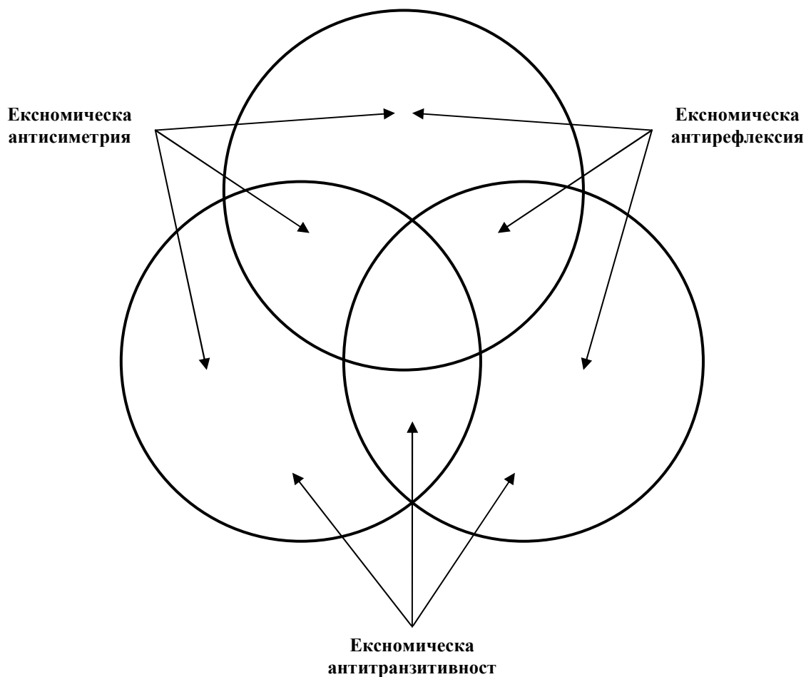
Фиг. 5.3. Видове на бинарно ексномическо отношение (трета част)
