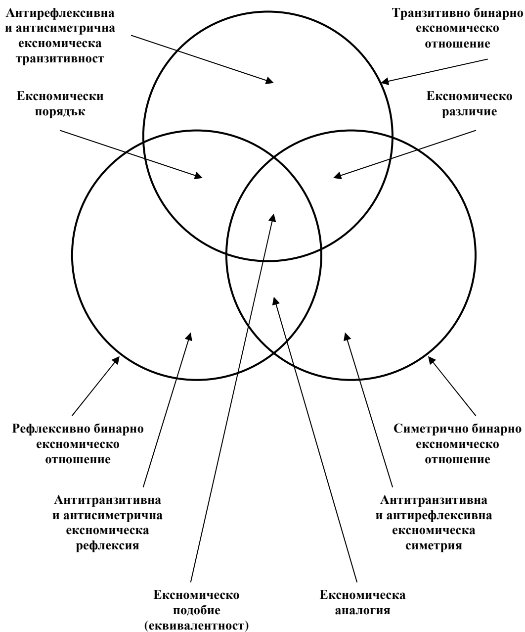
Фиг. 5.1. Видове на бинарно ексномическо отношение (първа част)
